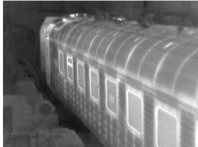
Рис. 1. Обследование кузова пассажирского вагона тепловизором при определении среднего коэффициента теплопередачи Fig. 1. Inspection of passenger car body with infrared imager for determination of the average heat transfer coefficient
